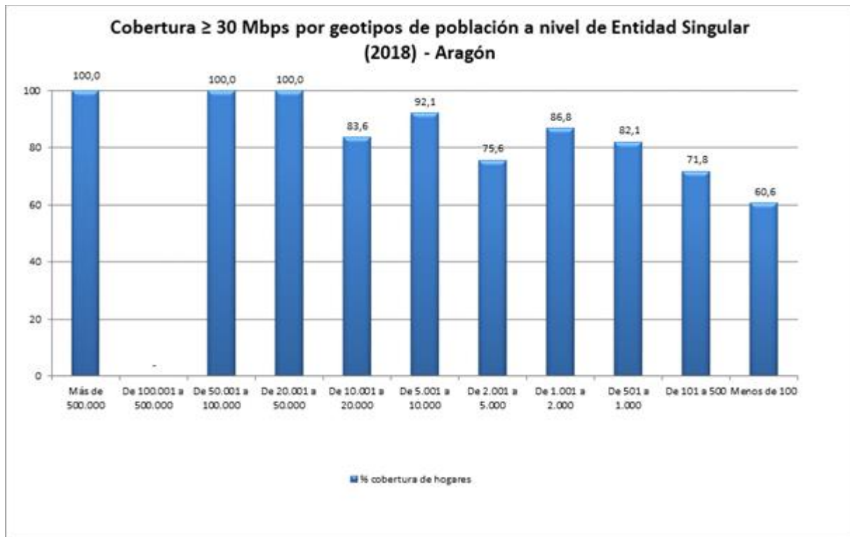
Ilustración 37.- Cobertura de redes fijas a velocidades \geq 30 Mbps por geotipo de población a nivel de entidad singular en Aragón a 30 de junio de 2018
