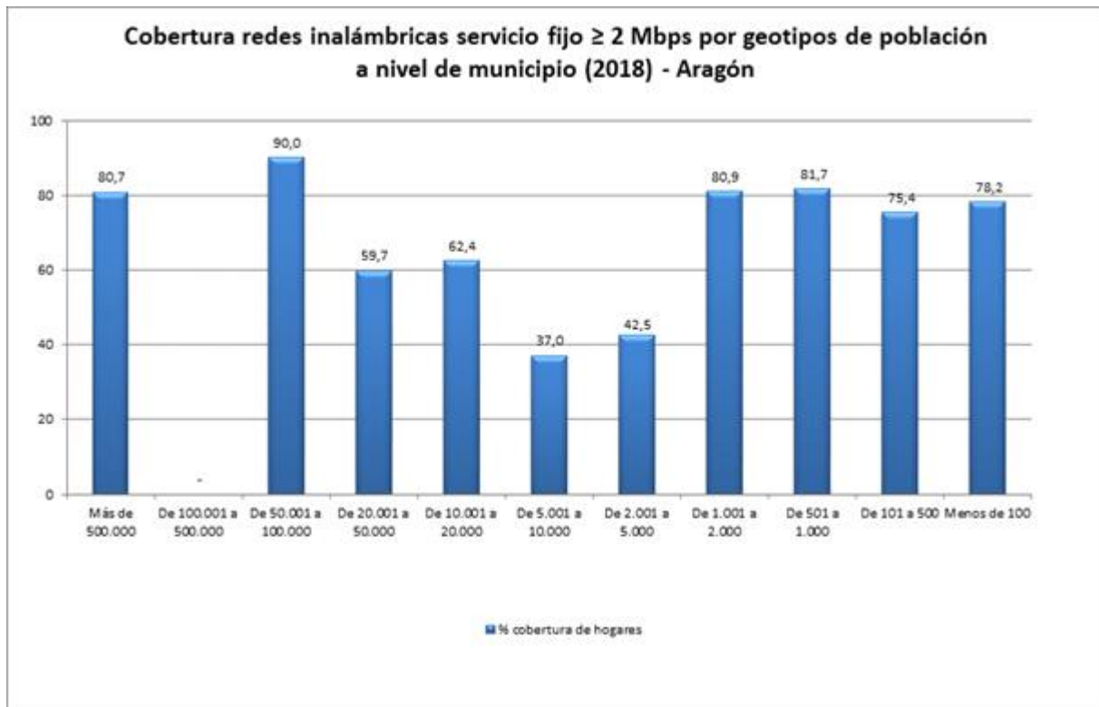
Ilustración 18.- Cobertura de redes inalámbricas servicio fijo \geq 2 Mbps por geotipo de población a nivel de municipio en Aragón a 30 de junio de 2018
