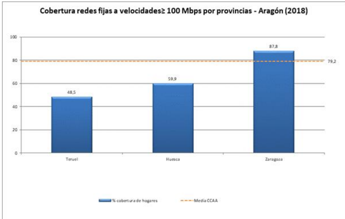
Ilustración 38.- Cobertura de redes fijas a velocidades \geq 100 Mbps por provincias en Aragón a 30 de junio de 2018
