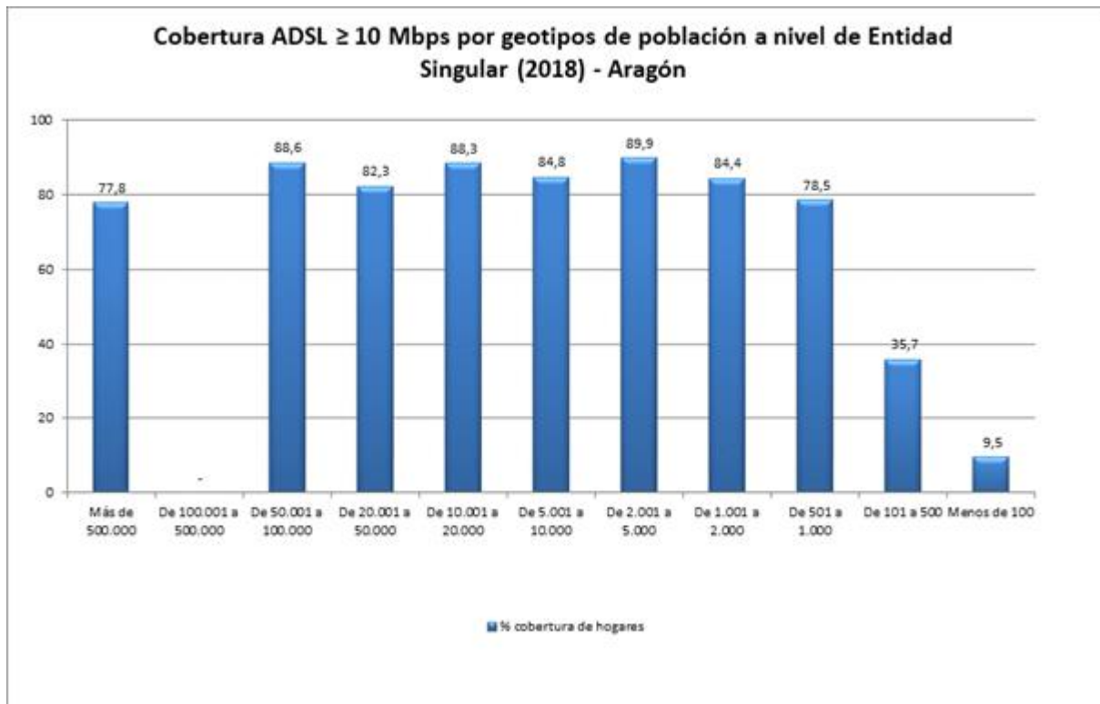
Ilustración 8.- Cobertura de ADSL ≥ 10 Mbps por geotipo de población a nivel de entidad singular en Aragón a 30 de junio de 2018
