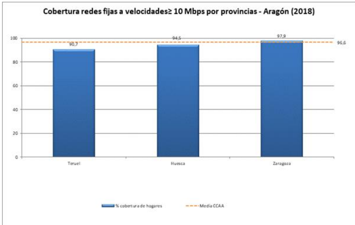
Ilustración 32.- Cobertura de redes fijas a velocidades \geq 10 Mbps por provincias en Aragón a 30 de junio de 2018
