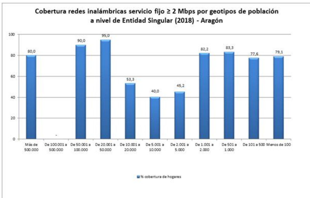
Ilustración 19.- Cobertura de redes inalámbricas servicio fijo \geq 2 Mbps por geotipo de población a nivel de entidad singular en Aragón a 30 de junio de 2018
