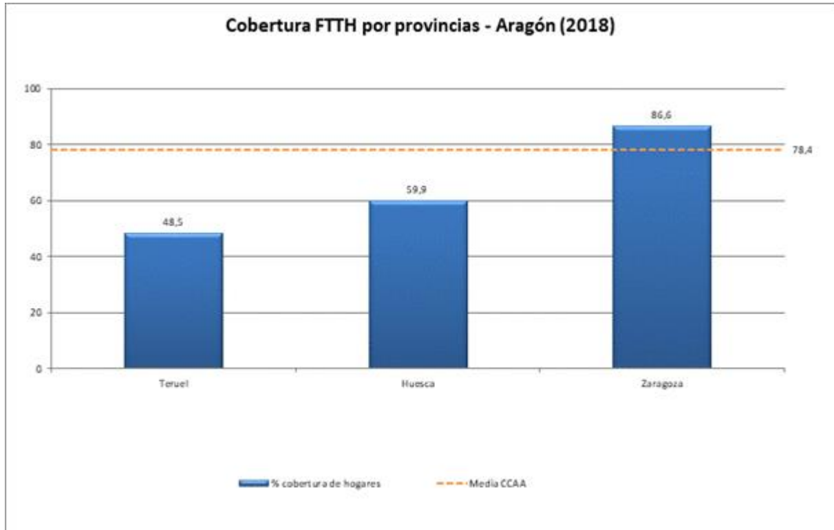
Ilustración 14.- Cobertura de FTTH por provincias en Aragón a 30 de junio de 2018
