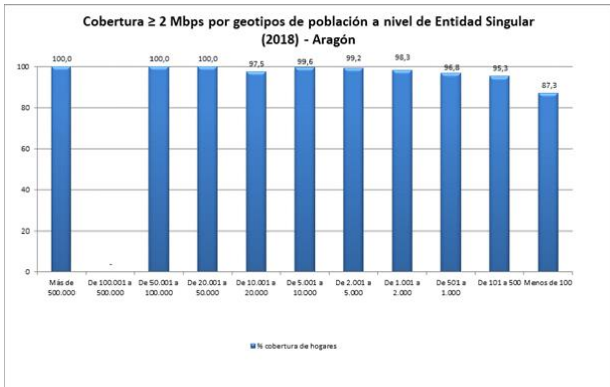
Ilustración 31.- Cobertura de redes fijas a velocidades \geq 2 Mbps por geotipo de población a nivel de entidad singular en Aragón a 30 de junio de 2018
