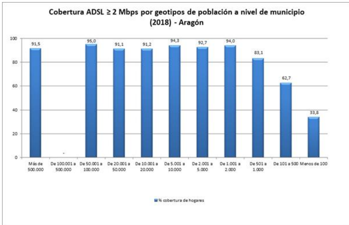
Ilustración 4.- Cobertura de ADSL \geq 2 Mbps por geotipo de población a nivel de municipio en Aragón a 30 de junio de 2018
